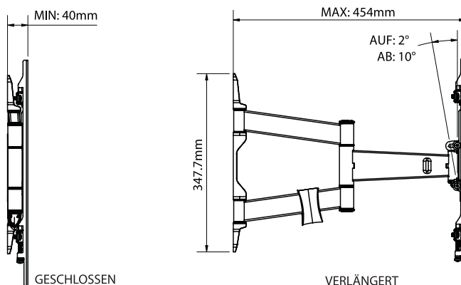
SEITENANSICHT
