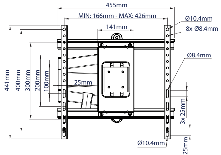
VORDERANSICHT
