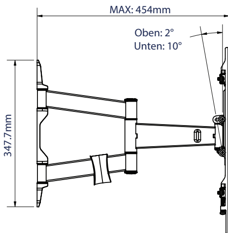
SEITENANSICHT - MAXIMALES AUSKLAPPEN
