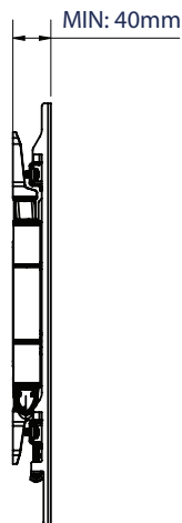
SEITENANSICHT - ARM FLACH AN DER WAND
