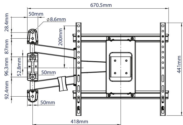
VORDERANSICHT MIT SEITLICH AUSGEKLAPPTEM ARM
