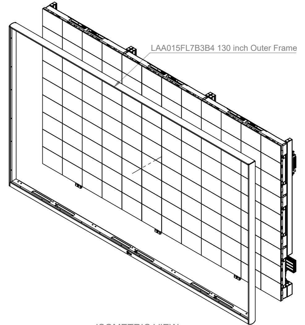
ISOMETRIC VIEW SCALE: 1 : 20
