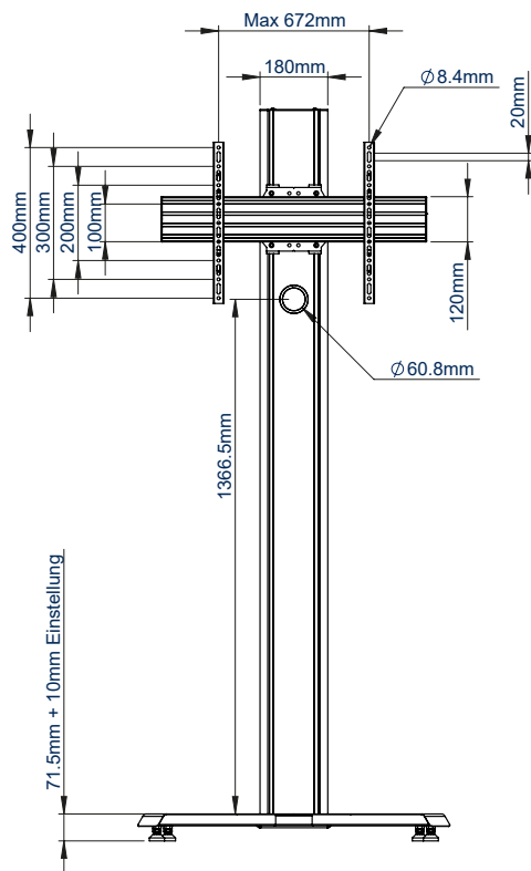
FRONTANSICHT
