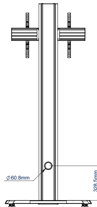
RÜCKANSICHT
