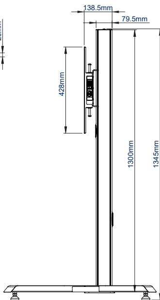
SEITENANSICHT
