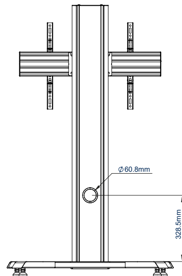
RÜCKANSICHT
