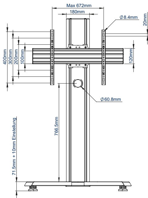
FRONTANSICHT
