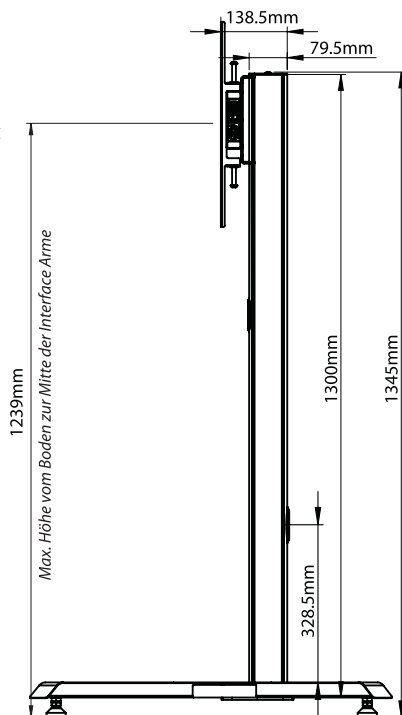
SEITENANSICHT
