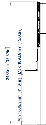
SEITENANSICHT
