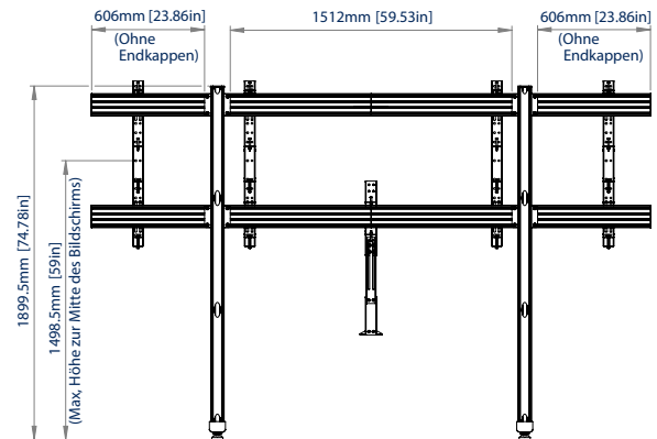
RÜCKANSICHT
