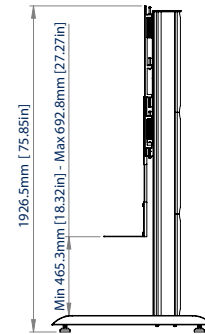
SEITENANSICHT
