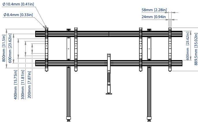
VORDERANSICHT
