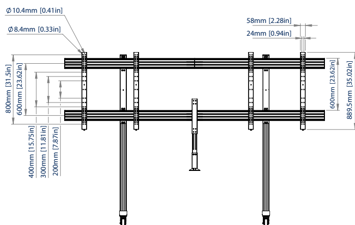
VORDERANSICHT
