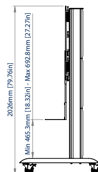
SEITENANSICHT
