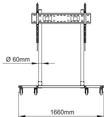
VORDERANSICHT
