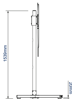
SEITENANSICHT MIT NIVELLIERFÜSSEN
