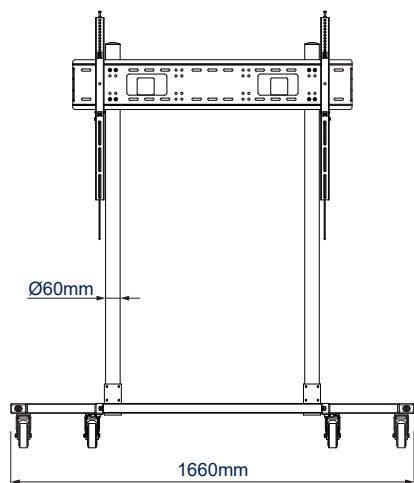
VORDERANSICHT MIT ROLLEN
