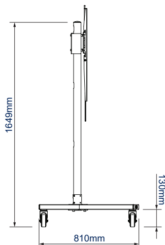
SEITENANSICHT MIT ROLLEN
