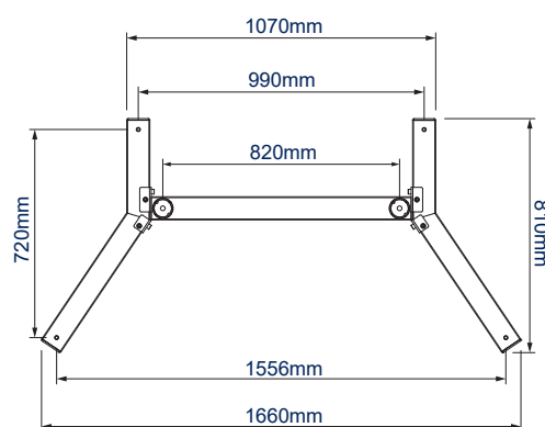
TROLLEY BASIS - ANSICHT VON OBEN
