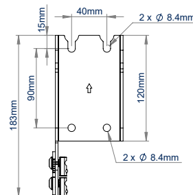
VORDERANSICHT
