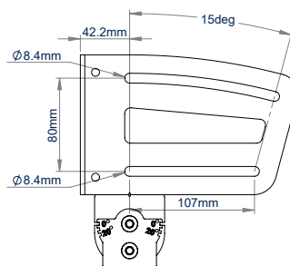
SEITENANSICHT
