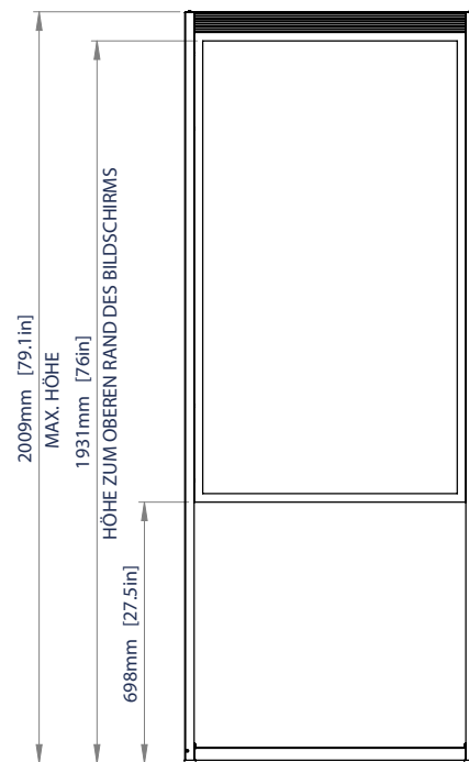
VORDERANSICHT
