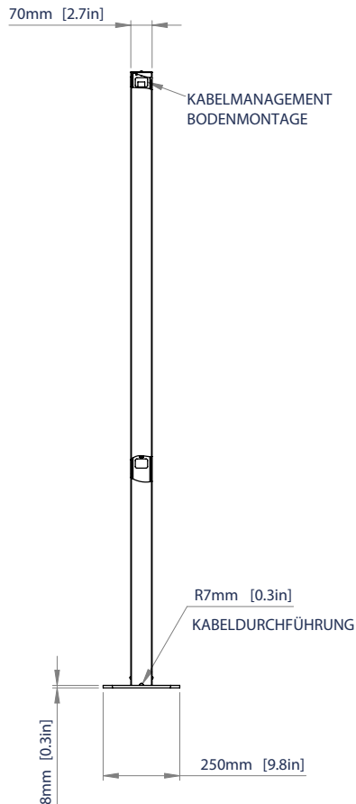
SEITENANSICHT
