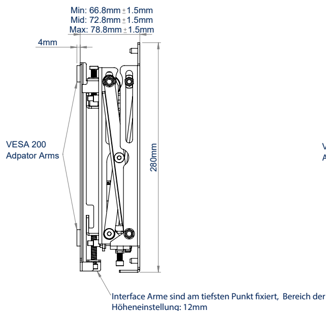
SEITENANSICHT GESCHLOSSEN
