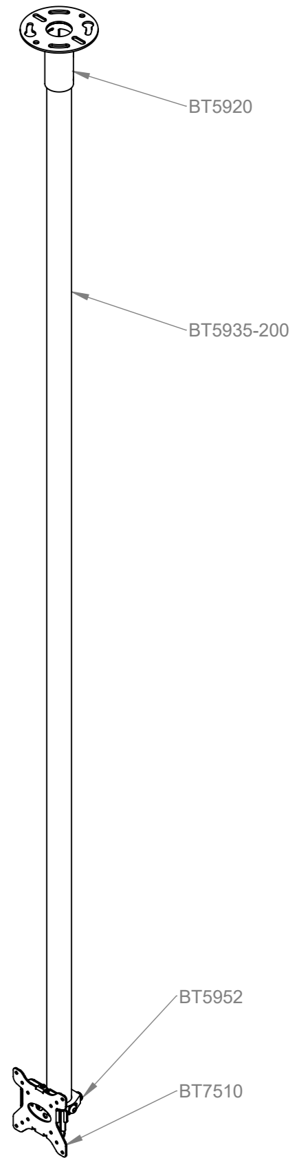
ISOMETRIC VIEW SCALE: 1 : 8
